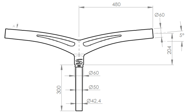
ELAYA TOP DOUBLE 480 / Pole Ø60
