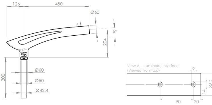
ELAYA TOP SIMPLE 480 / Pole Ø60
