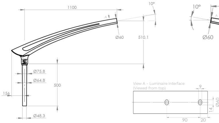
ELAYA TOP SIMPLE 1100 / Pole Ø76
